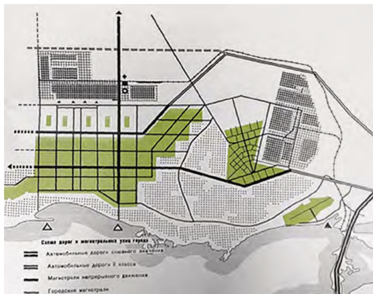
Схема генерального плана г. Тольятти, 1968–69 гг.
